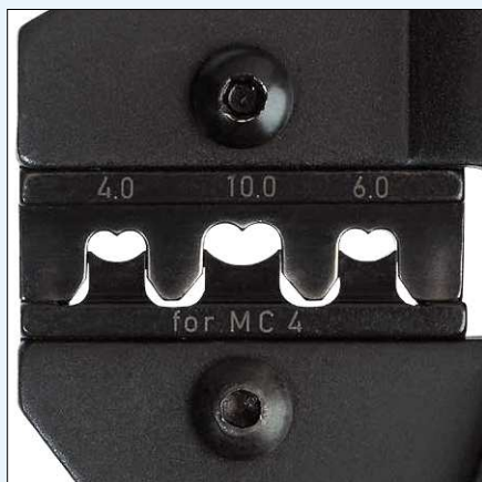
Crimpsenk, austauschbar (Anwendungsbeispiel für MC 4 - Verbinder)
