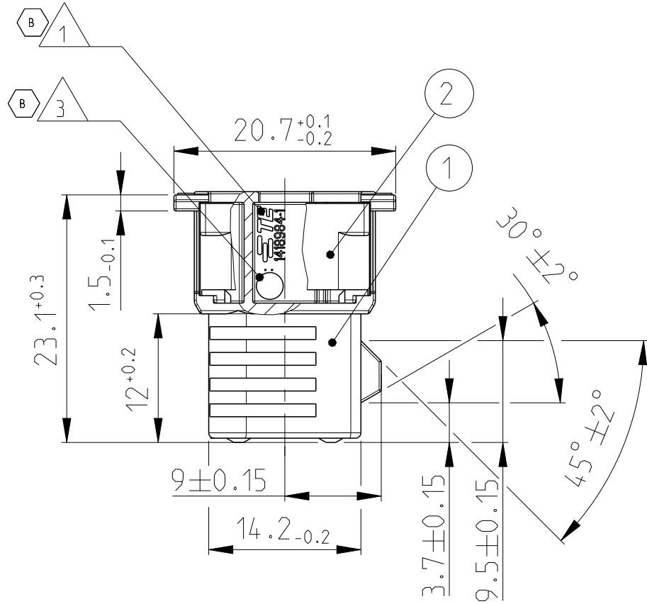
SECTION C-C Schnitt
