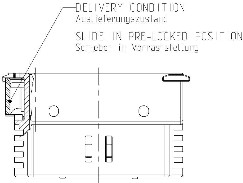
SECTION A-A Schnitt
