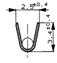
断面 C-C (SECT. C-C)
