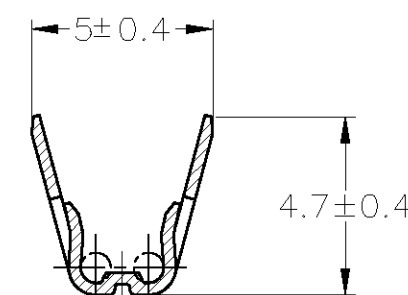
断面 B-B SECT B-B
