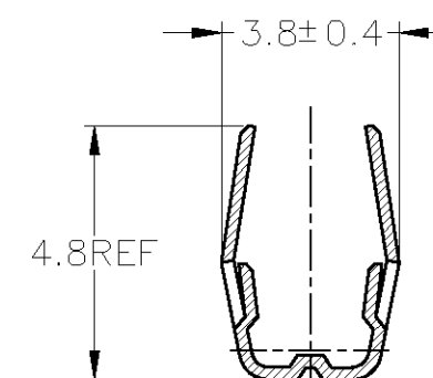
断面 B-B SECT B-B (175027のみ適用) (ONLY 175027)
